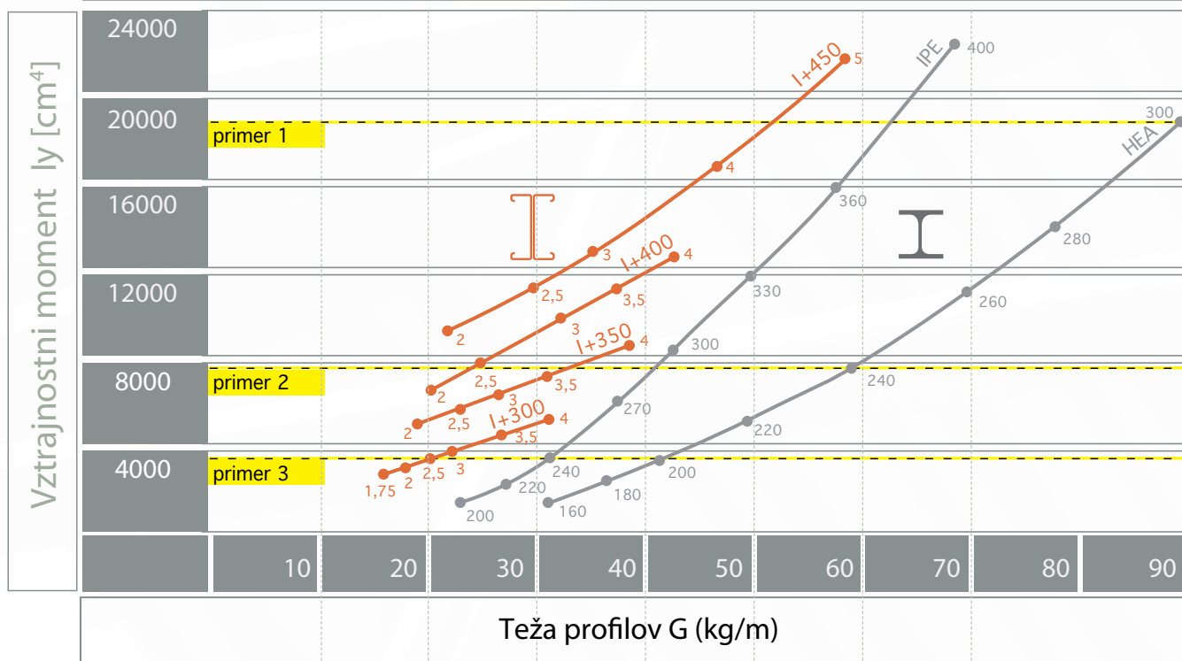
Prihranek na teži pri I-plus proti IPE/HEA profilom
