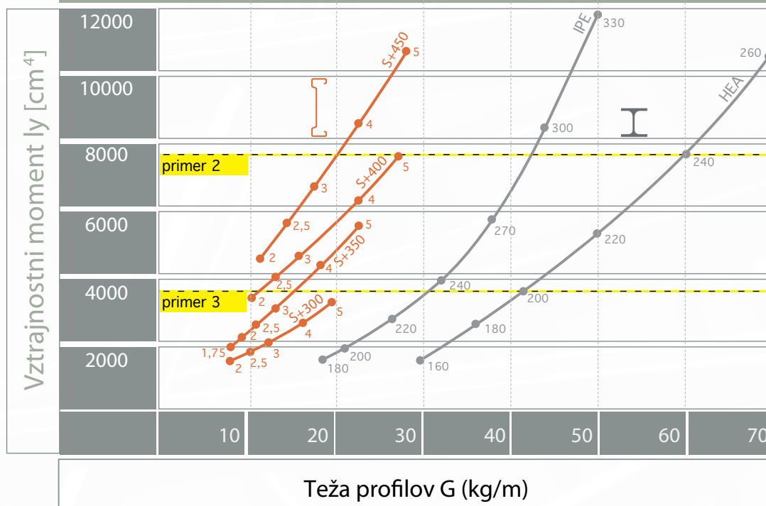
Prihranek na teži pri SIGMA- plus proti IPE/HEA profilom
